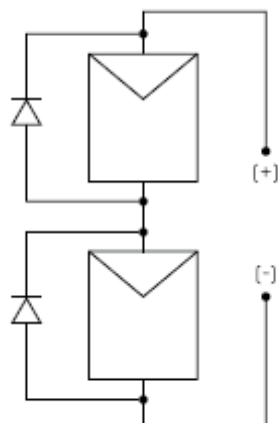
Figura: Diodos de desvio conectados em antiparalelo a cada módulo fotovoltaico
