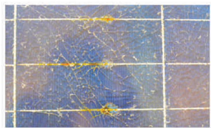
Figura: Célula fotovoltaica destruída por ponto quente.
