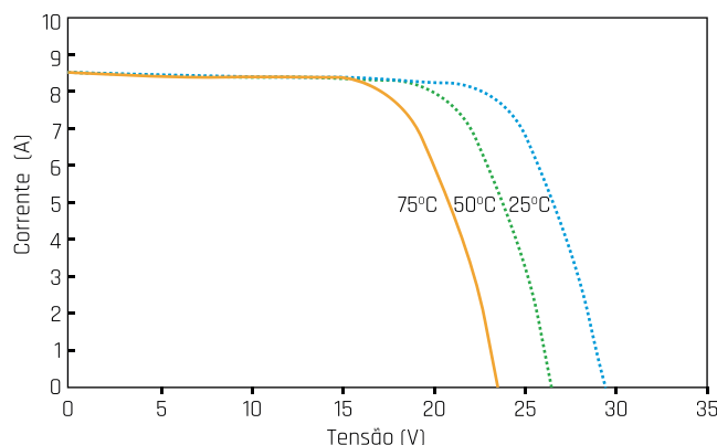
Figura: Curva I x V para diferentes temperaturas de células
