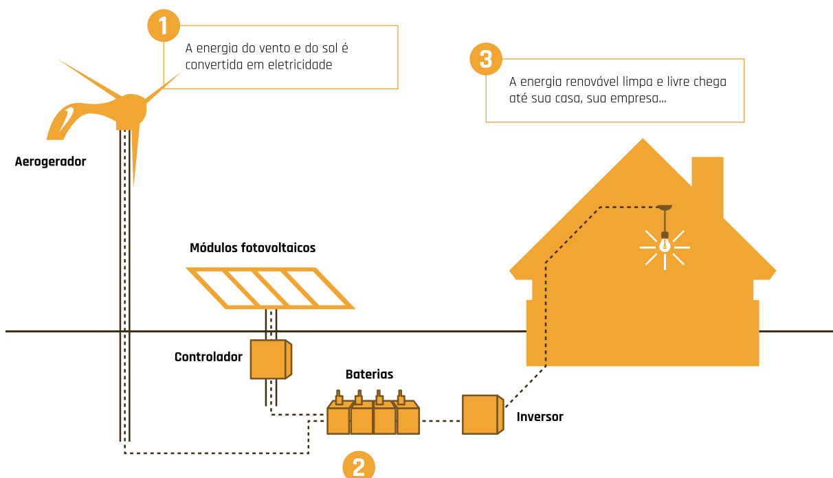
Figura: "Sistema Híbrido - Eólica Solar"
