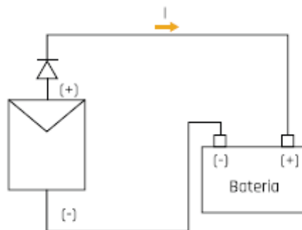
Figura: O diodo de bloqueio evita que a bateria injete corrente nos módulos durante a noite.
