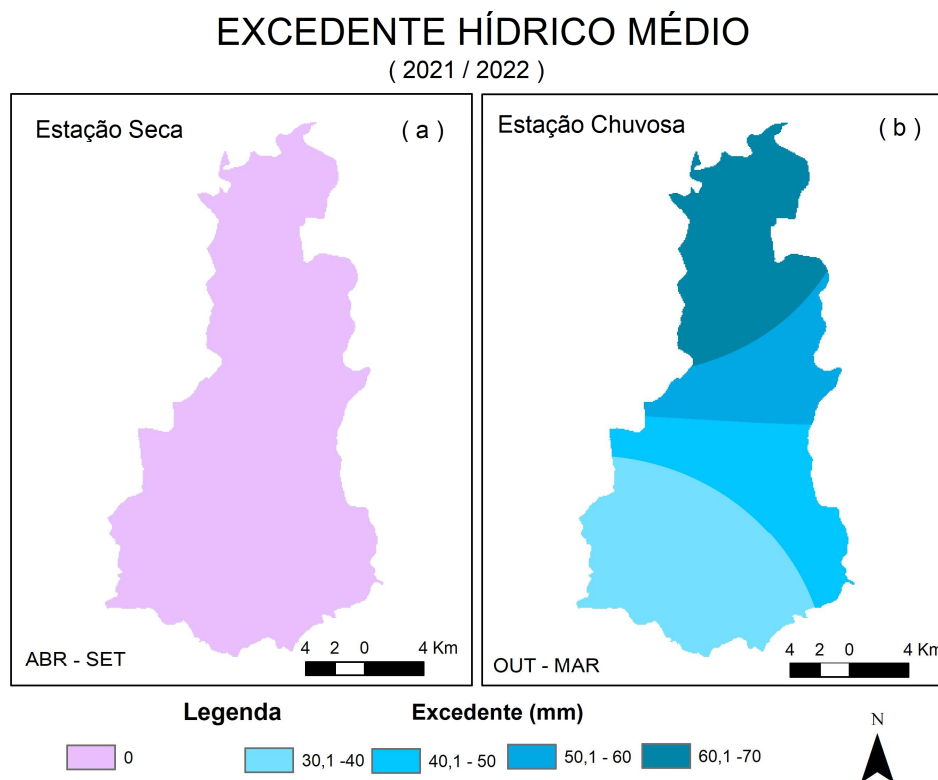
Figura 7: Espacialização da Excedente Hídrico Médio na Estação Seca (a) e na chuvosa (b) - (2021/2022). FONTE dos Dados: INMET e INPE
