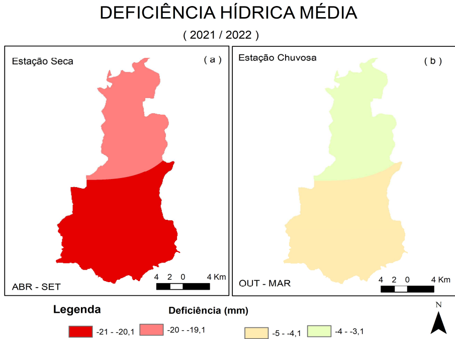
Figura 8: Espacialização da Deficiência Hídrica Média na Estação Seca (a) e chuvosa (b) - (2021/2022). FONTE dos Dados: INMET e INPE
