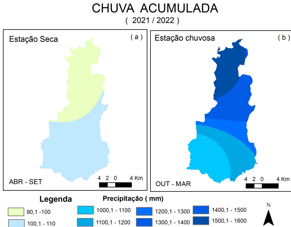
Figura 5: Espacialização da Chuva na Estação Seca (a) e chuvosa (b) - (2021/2022). FONTE dos Dados: INMET e INPE
