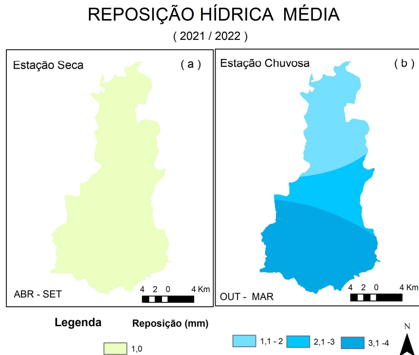
Figura 10: Espacialização da Reposição Hídrica Média na Estação Seca (a) e chuvosa (b) - (2021-2022). FONTE dos Dados: INMET e INPE
