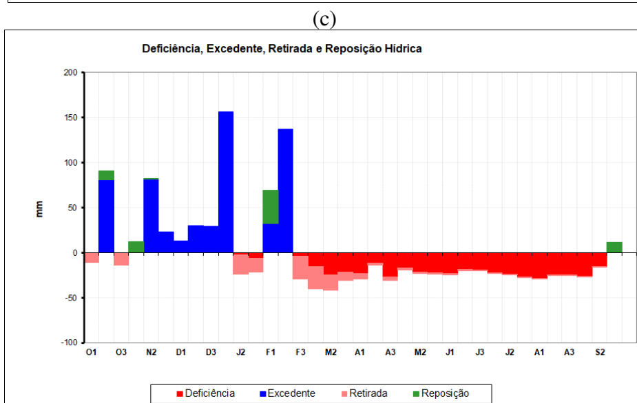
Figura 3: Balanços Hídricos: Caratinga(a); Timóteo (b) e PERD (c) – (2021/2022). FONTE dos Dados: INMET e INPE
