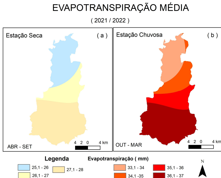
Figura 6: Espacialização da Evapotranspiração Média na Estação Seca (a) e chuvosa (b) - (2021/2022). FONTE dos Dados: INMET e INPE
