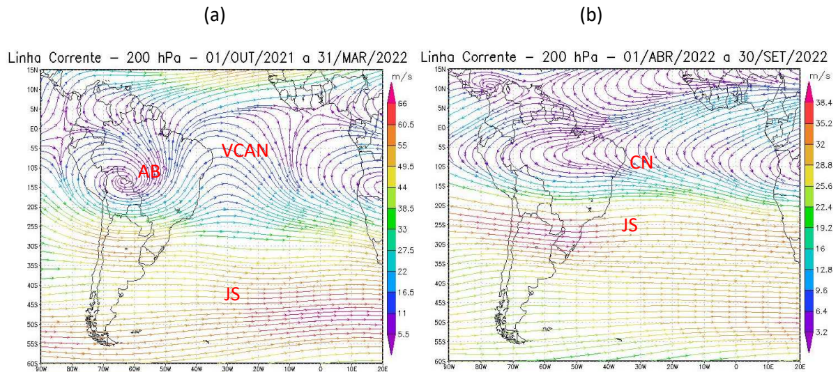
Figura 11: Campos de Linha de Corrente – Estação Seca - 200 hPa. (a) e Estação Chuvosa – 200 hPa (b); demonstrando interação entre os sistemas atmosféricos: Alta da Bolívia (AB), Vórtice Ciclônico de Altos níveis (VCAN), Cavado do Nordeste (CN) e Jato Subtropical (JS) - (2021/2022).
