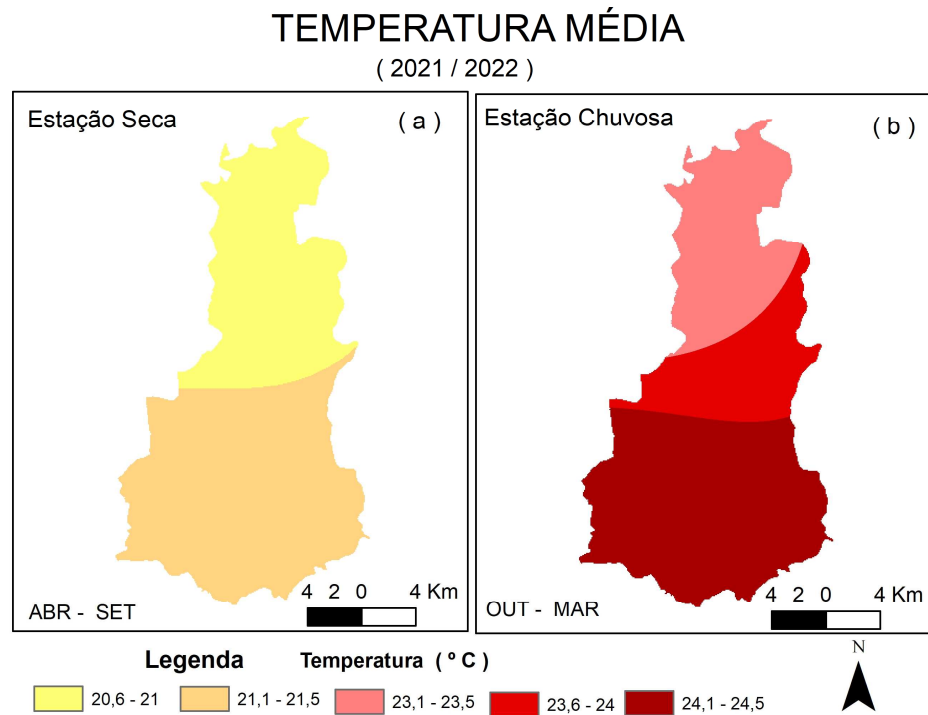
Figura 4: Espacialização da Temperatura Média na Estação Seca (a) e chuvosa (b) - (2021/2022). FONTE dos Dados: INMET e INPE
