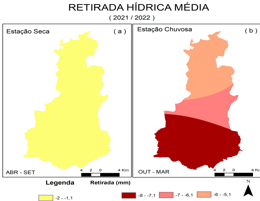
Figura 9: Espacialização da Retirada Hídrica Média na Estação Seca (a) e chuvosa (b) - (2021/2022). FONTE dos Dados: INMET e INPE
