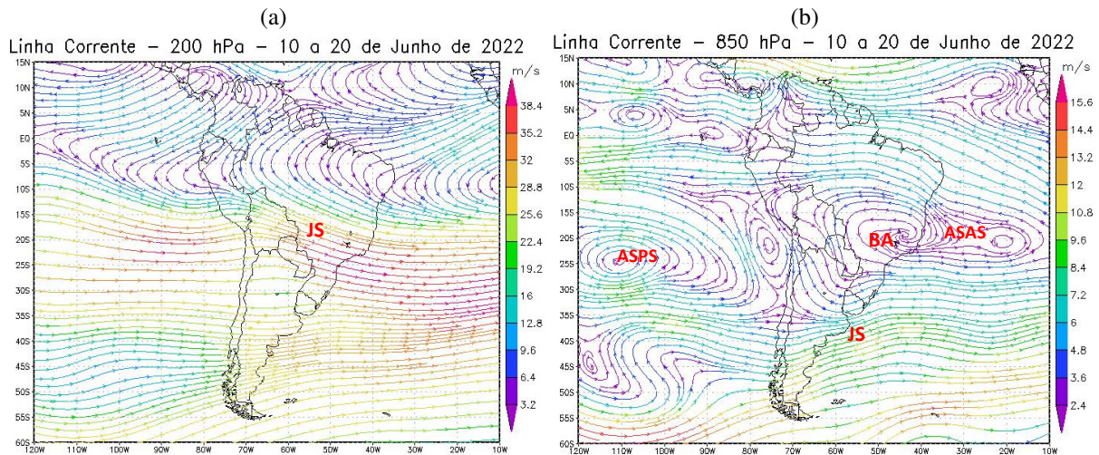
Figura 7 - Campos de Linha de Corrente 200 hPa. - (a) e 850 hPa. - (b), do 2º Decêndio de junho de 2022; demonstrando interação entre os sistemas atmosféricos: Jato Subtropical (JS), Bloqueio Atmosférico (BA), Anticiclone Subtropical do Atlântico Sul (ASAS) e o Anticiclone Subtropical do Pacífico Sul (ASPS). FONTE - Dados: NOAA 2022.
