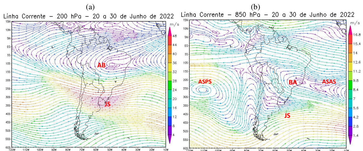
Figura 8 - Campos de Linha de Corrente 200 hPa. - (a) e 850 hPa. - (b), do 3º Decêndio de junho de 2022; demonstrando interação entre os sistemas atmosféricos: Alta da Bolívia (AB), Jato Subtropical (JS), Bloqueio Atmosférico (BA), Anticiclone Subtropical do Atlântico Sul (ASAS) e o Anticiclone Subtropical do Pacífico Sul (ASPS). FONTE - Dados: NOAA 2022.
