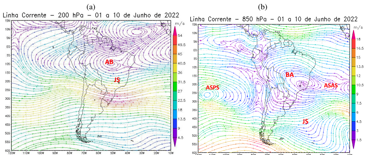
Figura 6 - Campos de Linha de Corrente 200 hPa. - (a) e 850 hPa. - (b), do 1º Decêndio de junho de 2022; demonstrando interação entre os sistemas atmosféricos: Jato Subtropical (JS), Alta da Bolívia (AB), Bloqueio Atmosférico (BA), Anticiclone Subtropical do Atlântico Sul (ASAS) e o Anticiclone Subtropical do Pacífico Sul (ASPS).
