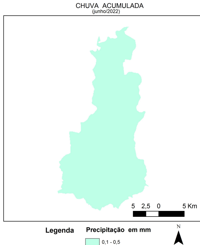
Figura 5 - Espacialização da Chuva da Acumulada em junho de 2022. FONTE dos Dados: INMET e INPE
