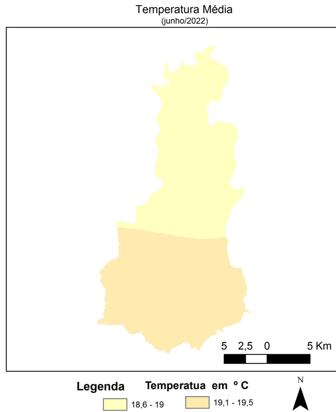
Figura 4 - Espacialização da Temperatura Média em junho de 2022. FONTE dos Dados: INMET e INPE
