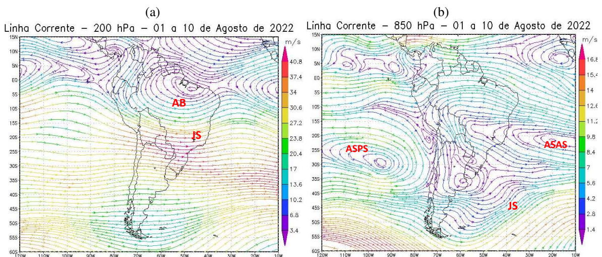
Figura 6 - Campos de Linha de Corrente 200 hPa. - (a) e 850 hPa. - (b), do 1º Decêndio de agosto de 2022; demonstrando interação entre os sistemas atmosféricos: Jato Subtropical (JS), Alta da Bolívia (AB), Anticiclone Subtropical do Atlântico Sul (ASAS) e o Anticiclone Subtropical do Pacífico Sul (ASPS).
