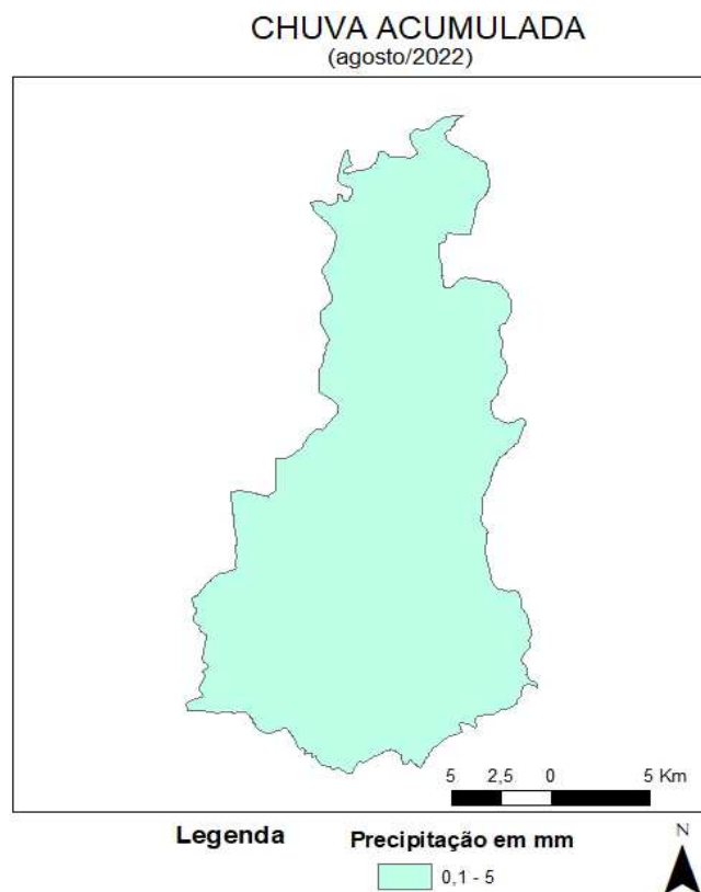
Figura 5 - Espacialização da Chuva da Acumulada em agosto de 2022. FONTE dos Dados: INMET e INPE
