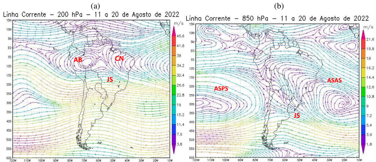
Figura 7 - Campos de Linha de Corrente 200 hPa. - (a) e 850 hPa. - (b), do 2º Decêndio de agosto de 2022; demonstrando interação entre os sistemas atmosféricos: Jato Subtropical (JS), Alta da Bolívia (AB) e Cavado do Nordeste (CN) Anticiclone Subtropical do Atlântico Sul (ASAS) e o Anticiclone Subtropical do Pacífico Sul (ASPS) .
