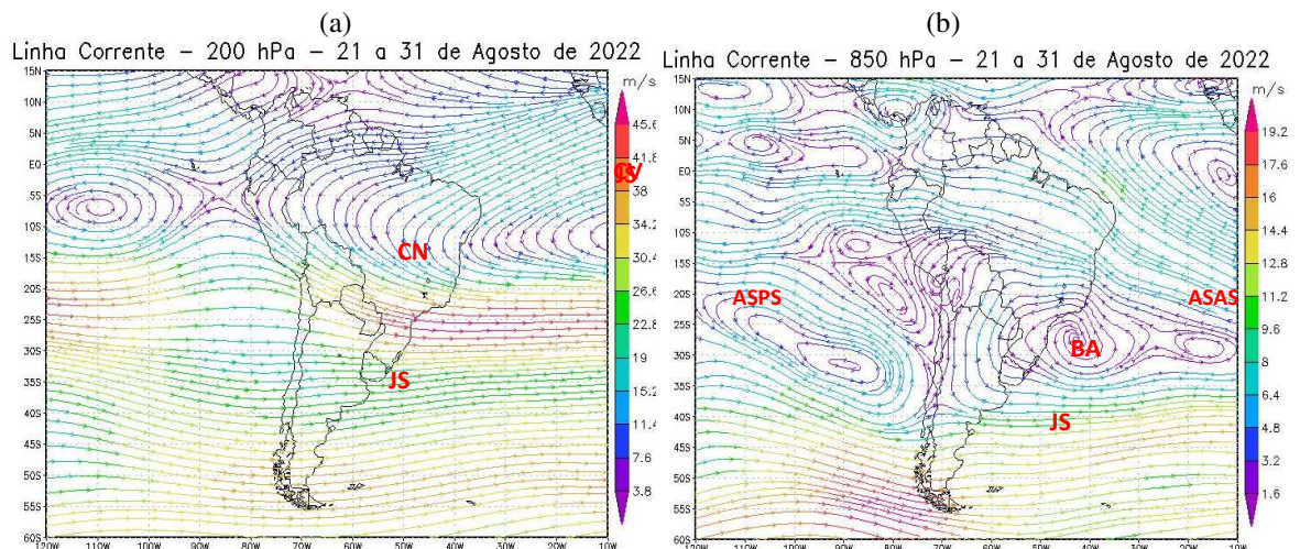
Figura 8 - Campos de Linha de Corrente 200 hPa. - (a) e 850 hPa. - (b), do 3º Decêndio de agosto de 2022; demonstrando interação entre os sistemas atmosféricos: Jato Subtropical (JS), Anticiclone Subtropical do Atlântico Sul (ASAS), Anticiclone Subtropical do Pacífico Sul (ASPS), Cavado do Nordeste (CN) e Bloqueio Atmosférico (BA)..
