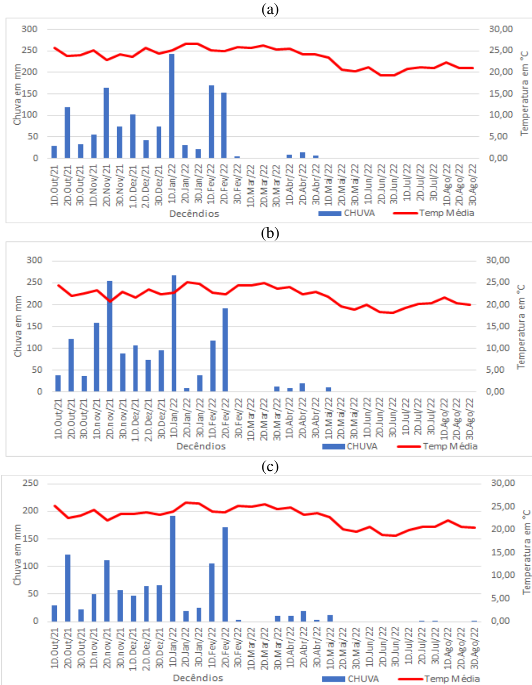
Figura 3: Histograma de Chuva e Temperatura: Caratinga (a); Timóteo (b) e PERD (c) – (outubro de 2021 a agosto de 2022).
