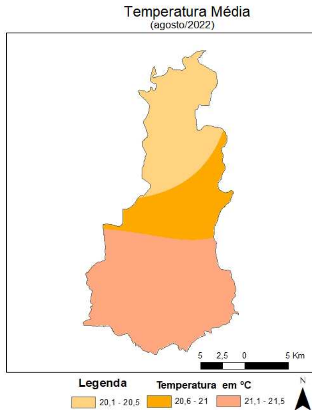
Figura 4 - Espacialização da Temperatura Média em agosto de 2022. FONTE dos Dados: INMET e INPE
