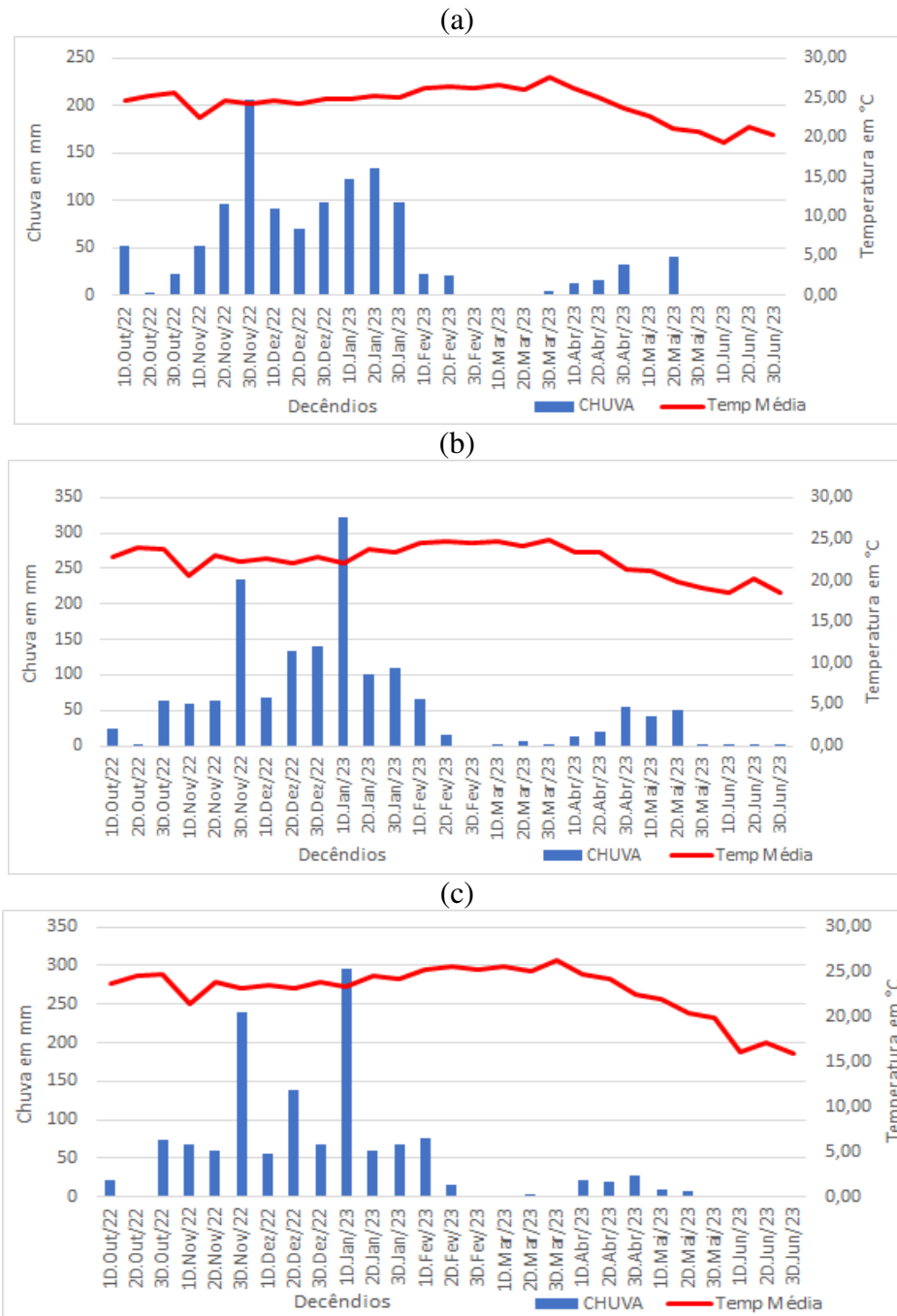
Figura 3: Histograma de Chuva e Temperatura: Caratinga (a); Timóteo (b) e PERD (c) – (outubro de 2022 a junho de 2023).
