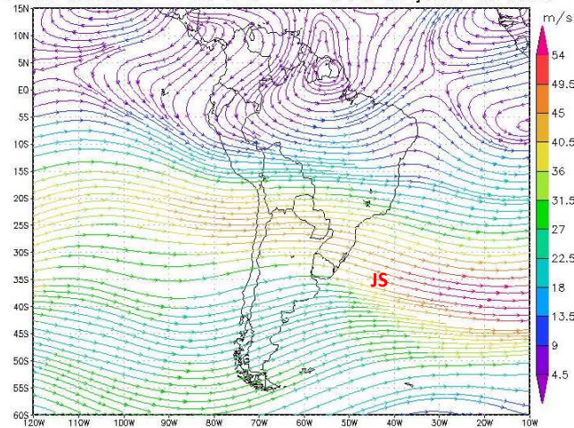
Linha Corrente – 500 hPa – 11 a 20 de junho de 2023
