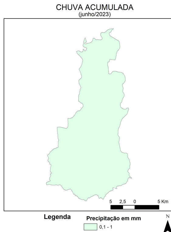
Figura 5 - Espacialização da Chuva da Acumulada em junho de 2023. FONTE dos Dados: INMET e INPE
