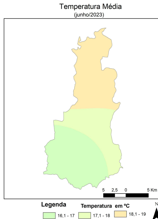
Figura 4 - Espacialização da Temperatura Média em junho de 2023. FONTE dos Dados: INMET e INPE
