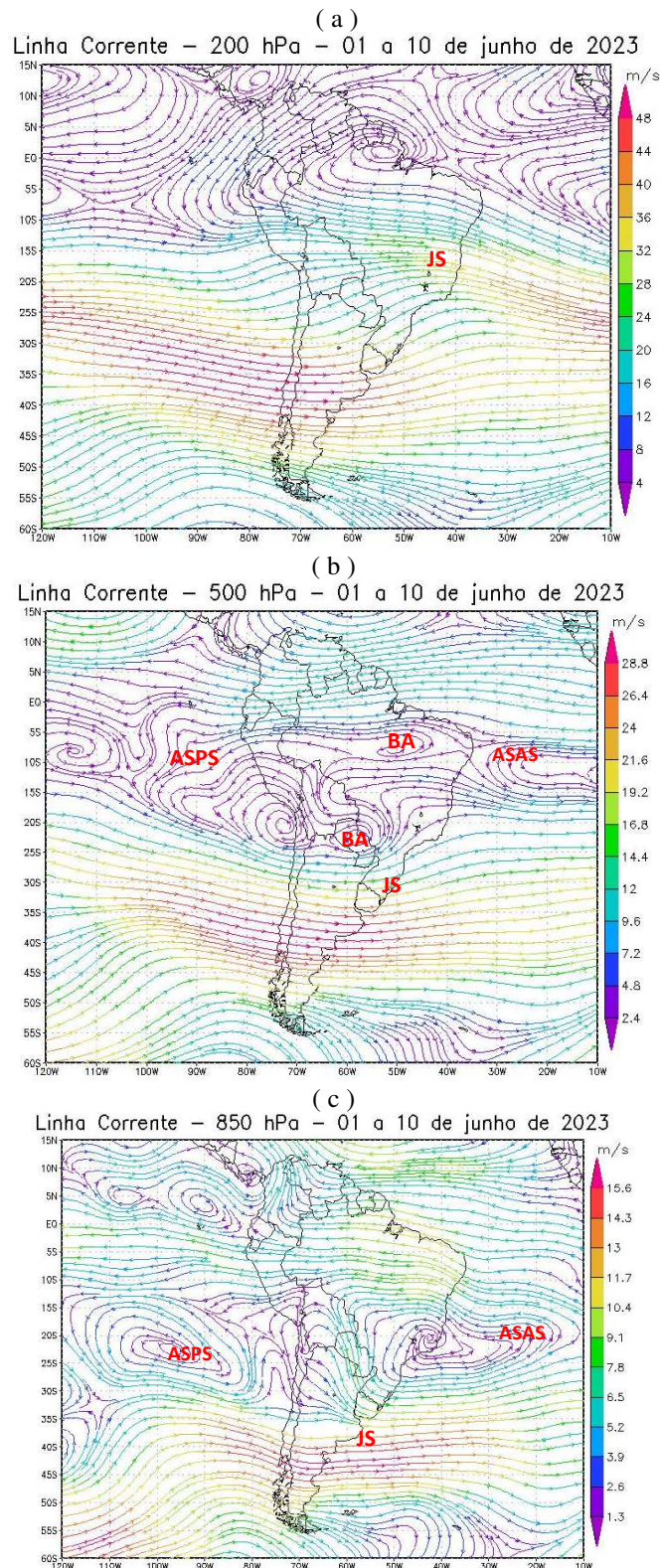
Figura 6 - Campos de Linha de Corrente 200 hPa - (a), 500 hPa - (b) e 850 hPa - (c), do 1º Decênio de junho de 2023; demonstrando interação entre os sistemas atmosféricos: Jato Subtropical (JS), Bloqueio Atmosférico (BA), Anticiclone Subtropical do Atlântico Sul (ASAS) e o Anticiclone Subtropical do Pacífico Sul (ASPS). FONTE - Dados: NOAA 2023.
