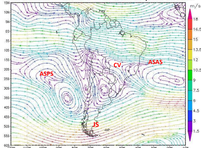
Figura 7 - Campos de Linha de Corrente 200 hPa - (a), 500 hPa - (b) e 850 hPa - (c), do 2º Decêndio de junho de 2023; demonstrando interação entre os sistemas atmosféricos: Jato Subtropical (JS), Bloqueio Atmosférico (BA), Cavado (CV), Anticiclone Subtropical do Atlântico Sul (ASAS) e o Anticiclone Subtropical do Pacífico Sul (ASPS).
