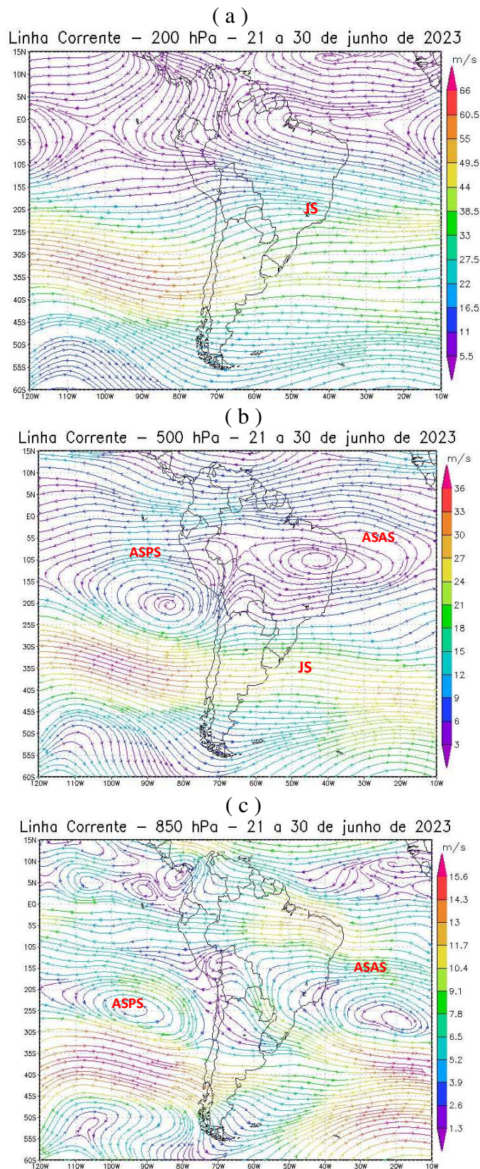
Figura 8 - Campos de Linha de Corrente 200 hPa- (a), 500 hPa- (b) e 850 hPa – (c), do 3º Decêndio de junho de 2023; demonstrando interação entre os sistemas atmosféricos: Jato Subtropical (JS), Anticiclone Subtropical do Atlântico Sul (ASAS) e Anticiclone Subtropical do Pacífico Sul (ASPS).
