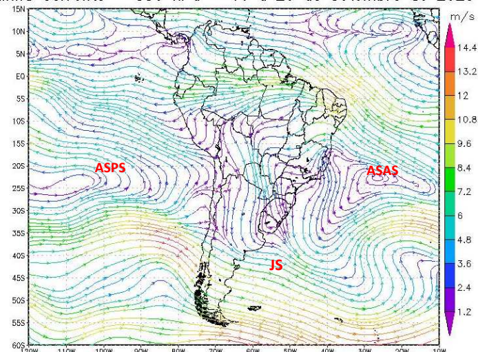
Figura 7 - Campos de Linha de Corrente 200 hPa (a), 500 hPa (b) e 850 hPa (c), do 2º Decêndio de setembro de 2025; demonstrando interação entre os sistemas atmosféricos: Jato Subtropical (JS), Anticiclone Subtropical do Atlântico Sul (ASAS) e o Anticiclone Subtropical do Pacífico Sul (ASPS).
