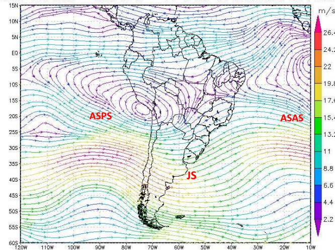
(c) Linha Corrente – 850 hPa – 11 a 20 de Setembro de 2025
