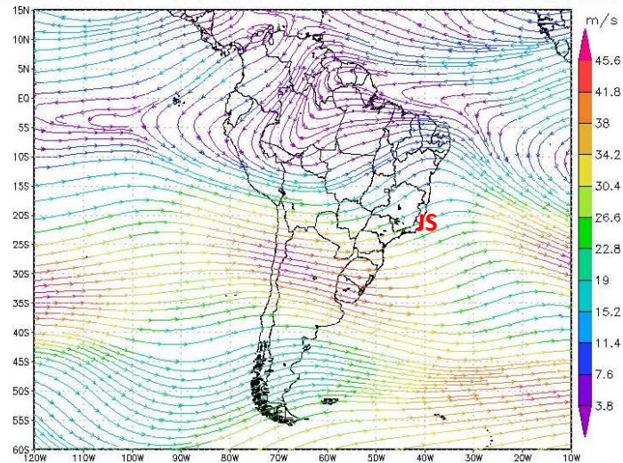
(b) Linha Corrente – 500 hPa – 01 a 10 de Setembro de 2025
