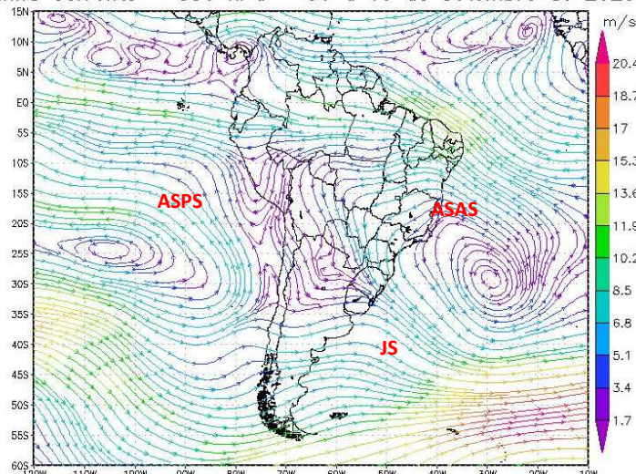
Figura 6 - Campos de Linha de Corrente 200 hPa (a), 500 hPa (b) e 850 hPa (c), do 1º Decêndio de setembro de 2025; demonstrando interação entre os sistemas atmosféricos: Jato Subtropical (JS), Alta da Bolívia, Anticiclone Subtropical do Atlântico Sul (ASAS) e o Anticiclone Subtropical do Pacífico Sul (ASPS).
