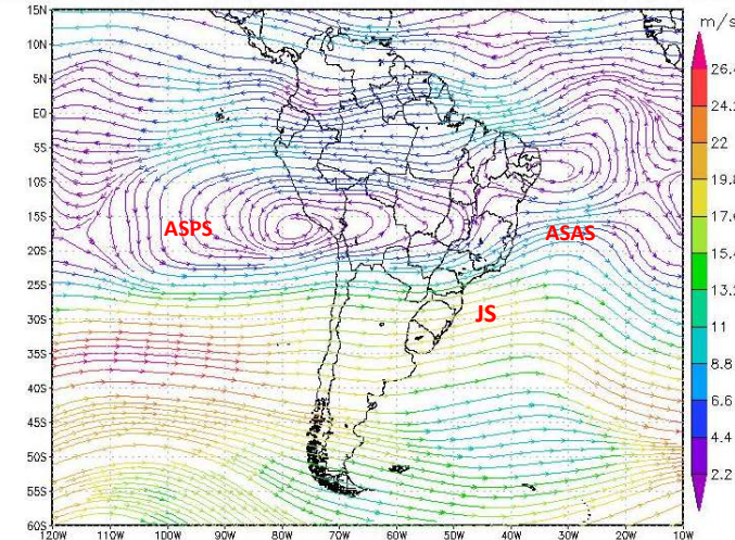
(c) Linha Corrente – 850 hPa – 21 a 30 de Setembro de 2025
