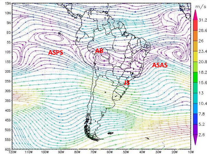
(c) Linha Corrente – 850 hPa – 01 a 10 de Setembro de 2025
