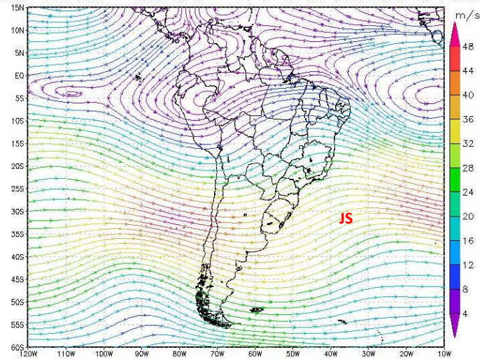
(b) Linha Corrente – 500 hPa – 11 a 20 de Setembro de 2025
