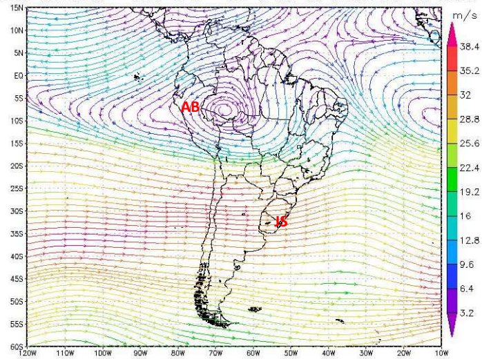
(b) Linha Corrente – 500 hPa – 21 a 30 de Setembro de 2025
