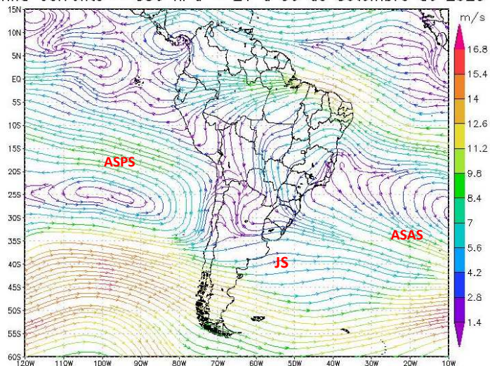
Figura 8 - Campos de Linha de Corrente 200 hPa (a), 500 hPa (b) e 850 hPa (c), do 3º Decêndio de setembro de 2025; demonstrando interação entre os sistemas atmosféricos: Jato Subtropical (JS), Alta da Bolívia, Anticiclone Subtropical do Atlântico Sul (ASAS) e Anticiclone Subtropical do Pacífico Sul (ASPS).
