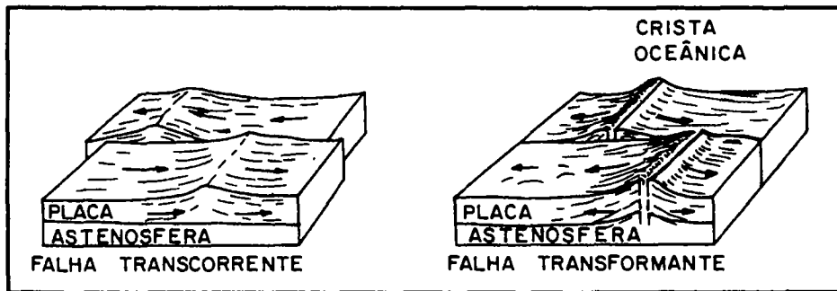
Fig. 3.11. Tipos de falhas deslizantes.
