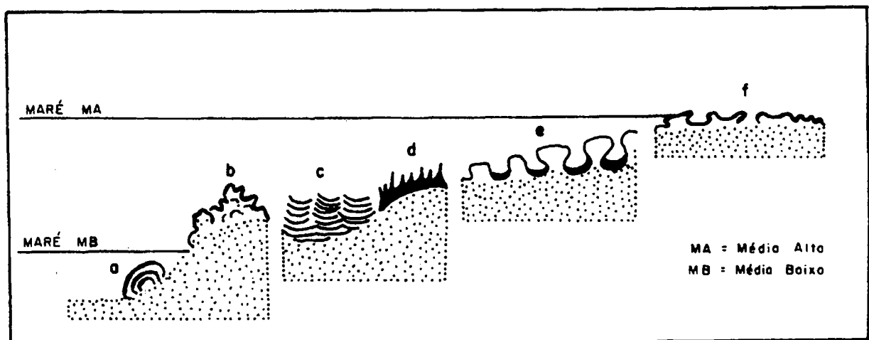
Fig. 4.3. Seqüência moderna da localização dos tipos de tapete algal na zona de intermaré no Golfo Pérsico. Adaptado de Golubic (em Walter, 1976).
