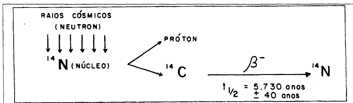
Fig. 2.6. Esquema da formação do isótopo radioativo de carbono (C-14).
