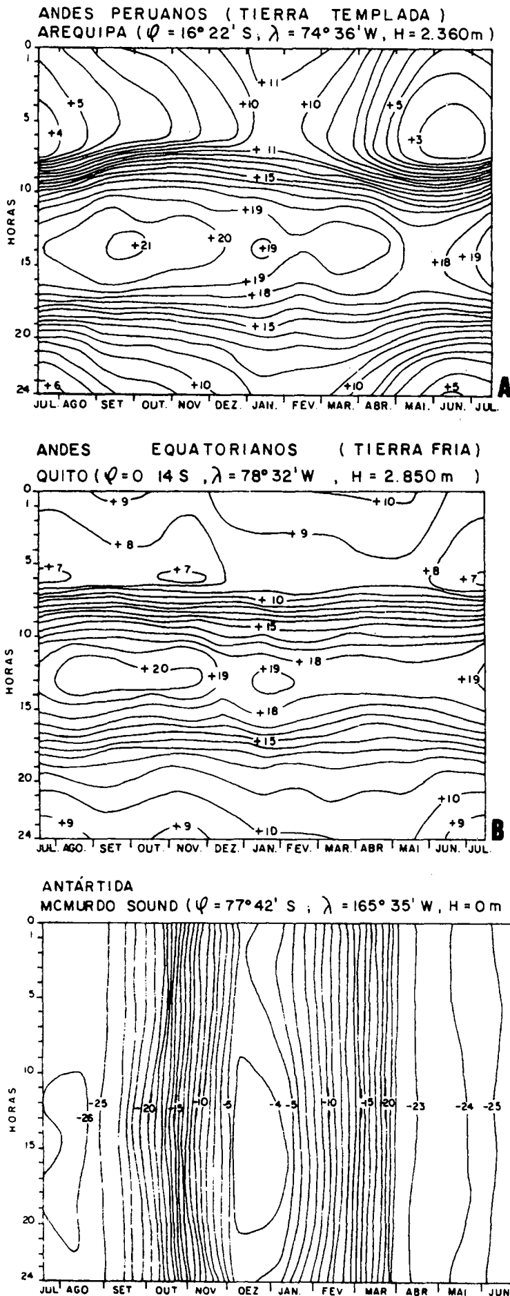
Fig. 8.4. Três exemplos de termoisopletes que caracterizam os climas temperados e frios: A. temperado de alta montanha; B. frio de alta montanha; C. frio da zona polar antártica. Adaptado de Troll (1972). Nesta representação as linhas isopletes se desenvolvem na horizontal nas altas montanhas tropicais (A e B) caracterizando dias quentes e noites frias o ano todo; elas se desenvolvem na vertical (C) na zona antártica (nos climas temperados) onde meses mais ou menos frios caracterizam as estações do ano.
