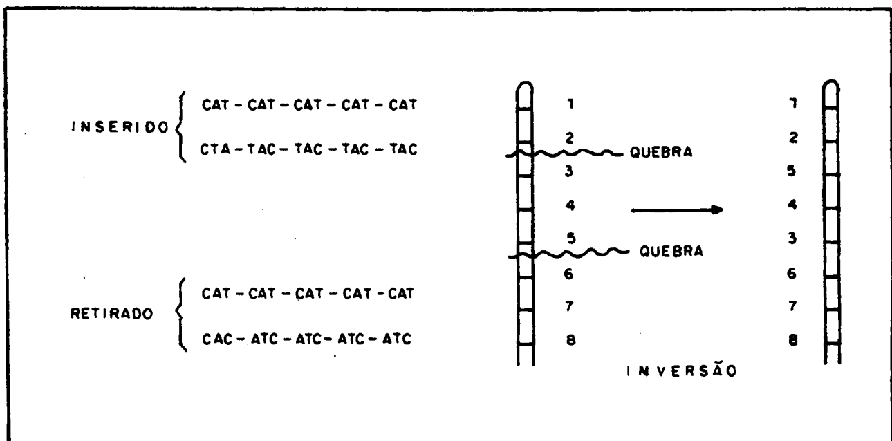
Fig. 5.14. Exemplos de mutações por adição (inserido), deleção (retirado) e inversão na seqüência de nucleotídeos do cromossomo.
