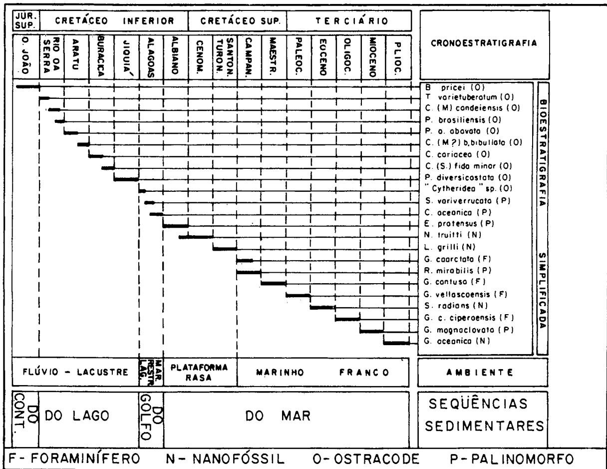
Fig 5.6. Seqüência cronológica da ocorrência de microfósseis na plataforma continental brasileira que mostra a formação do Atlântico Sul. O conjunto de microfósseis (assemblage) passa de continental a marinho ao longo do tempo. Segundo Viana (1980).
