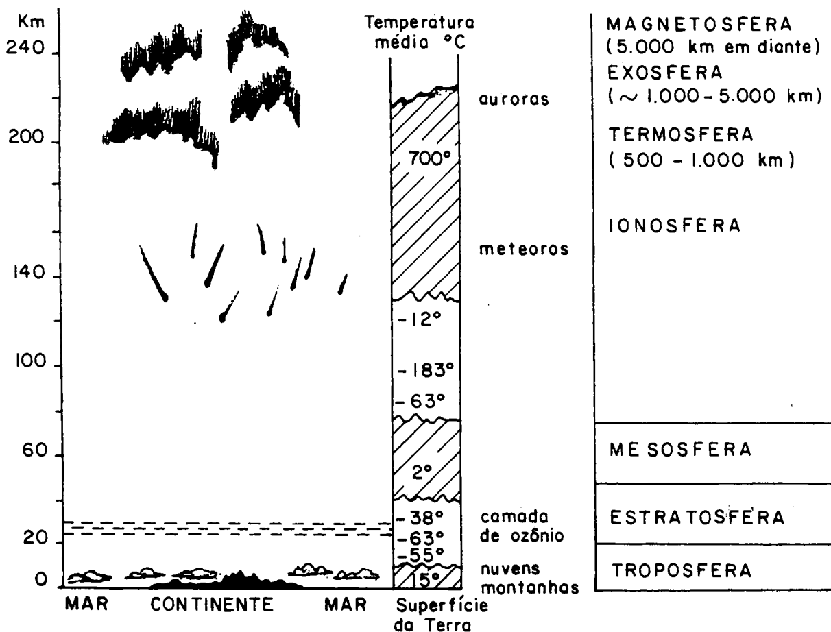
Fig. 7.5. A atmosfera pode ser dividida em 7 camadas (á direita da figura) que não têm limites altitudinais precisos e que passam de uma camada à outra gradualmente. As camadas superiores (termosfera, ionosfera e magnetosfera) não estão em escala.
