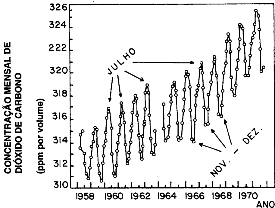
Fig. 7.8. Primeiras medidas do aumento da concentração média mensal de dióxido de carbono registradas na atmosfera em Mauna Loa, Havaí, durante 14 anos, segundo L. Machta (em Rosenberg, 1974 e Ingersoll, 1983).
