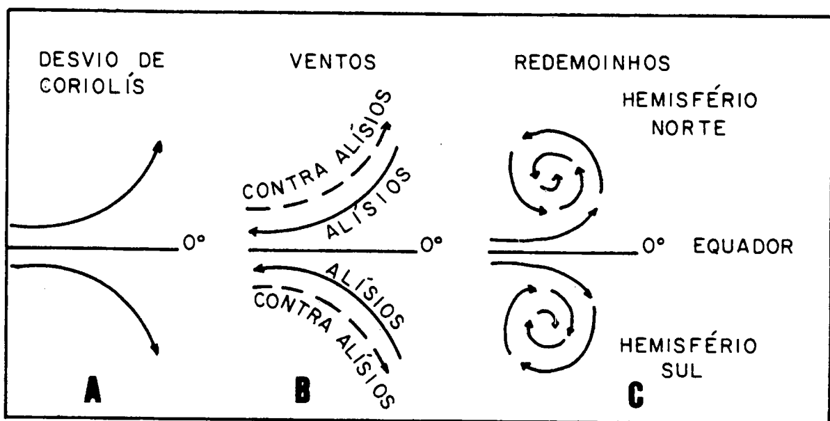
Fig. 8.9. Alguns efeitos devidos à aceleração de Coriolis. A: desvio na direção das massas de ar que se originam na zona equatorial; B: movimento das massas de ar superficial que vêm da zona sub-tropical para o equador; C: sentido direcional dos redemoinhos em cada um dos hemisférios da Terra.
