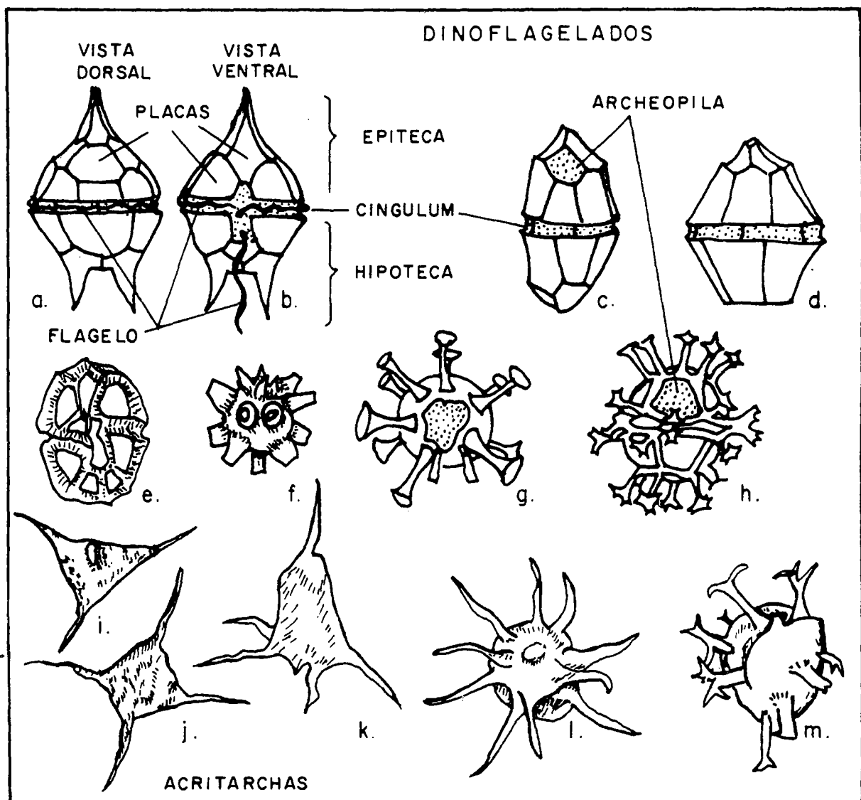
Fig. 4.8. Em cima e no meio: Dinoflagelados (Pyrrhophyta, classe Dinophyceae) com carapaça externa de esporopolenina; a e b : forma moderna, móvel, de Peridinales com dois flagelos; c ao h : vários tipos de cistos do Mesozóico ao Presente. Em baixo, i ao m : vários tipos de carapaças de esporopolenina de Acritarcas do Paleozóico do Canadá (Evitt, 1985 e artigos no periódico "Palynology" vol. 9, 1985).
