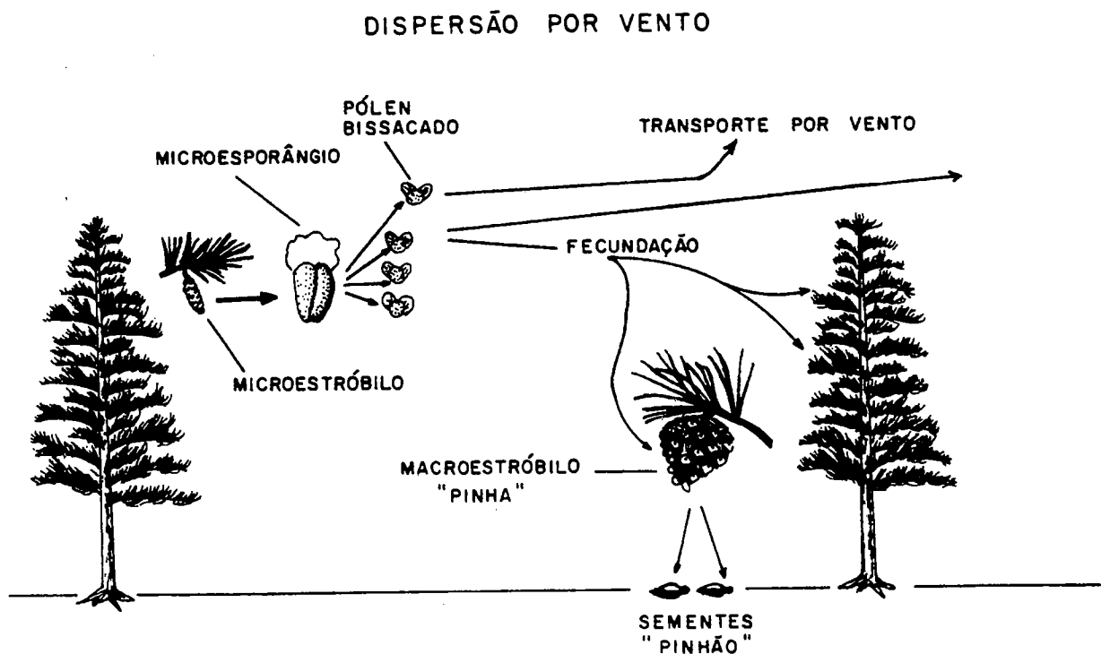
Fig. 5.7. O vetor de polinização em uma conífera é o vento (anemofilia). O pólen produzido em uma árvore é levado pelo vento até o cone feminino ou pinha (macroestróbilo) de outra árvore; aí se dá a fecundação e a formação da semente (pinhão); cada grão de pólen tem um, dois ou três sacos cheios de ar (conforme a espécie) que permitem maior flutuação no ar; nesta representação o pólen é bi-sacado. A maior parte do pólen dispersado pelo vento cai na superfície do solo ou da água, onde pode ser incorporado ao sedimento, ficando preservado como fóssil.
