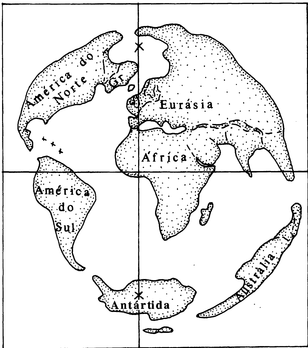
Fig. 6.8. Posição dos continentes no Mioceno inferior, em relação ao equador e o meridiano de Greenwich. A forma dos continentes é somente como referência, mas já se aproxima da moderna. O x marca os polos sul e norte.
