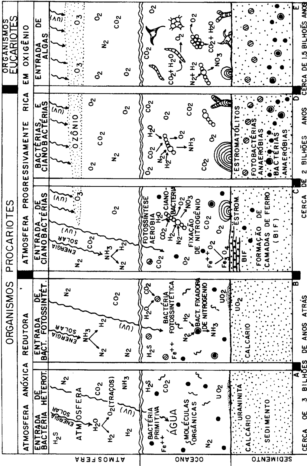
Fig. 7.10 Esquema da evolução do ambiente na atmosfera, no mar e nos sedimentos marinhos entre 3 bilhões e 1,5 bilhões de anos atrás. A - Arqueano, desenvolvimento das primeiras bactérias anaeróbias no mar; B - surgimento das bactérias fotossintéticas e das fixadoras de nitrogênio, que trouxeram uma mudança química no ar e no mar; C - desenvolvimento das cianobactérias no mar e início da acumulação de oxigênio que resultou na formação de espessas camadas de óxido de ferro (BIF); D - acumulação de oxigênio em quantidades apreciáveis no oceano e na atmosfera que deslocou as bactérias anaeróbias para o ambiente anóxico dos sedimentos marinhos; E - desenvolvimento de outros organismos marinhos; a camada de ozônio da atmosfera está completa. Esquema baseado em Schopf (1978).
