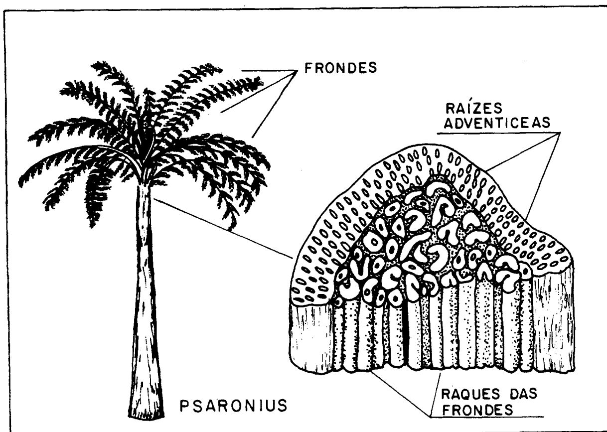
Fig. 4.13. Reconstrução de uma planta de Psaronius , que mostra ser ela um feto arborescente (samambaiáçu). À direita, um corte transversal da região onde os raquis das folhas (frondes) se comprimem. Desenho baseado em um exemplar fóssil encontrado por M. Dardenne em Filadélfia, estado do Maranhão, Brasil.
