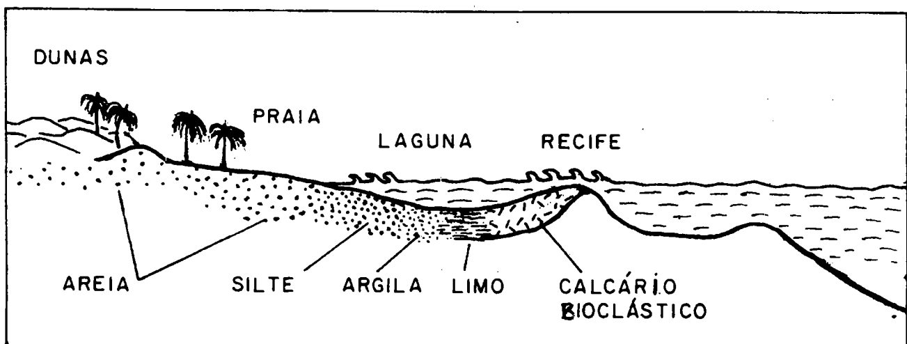
Fig. 9.13. Esquema de um litoral com recife e formação de laguna. Os sedimentos do piso oceânico se dispõem em gradação desde partículas maiores (areia) na praia, até a lama muito fina, na laguna.
