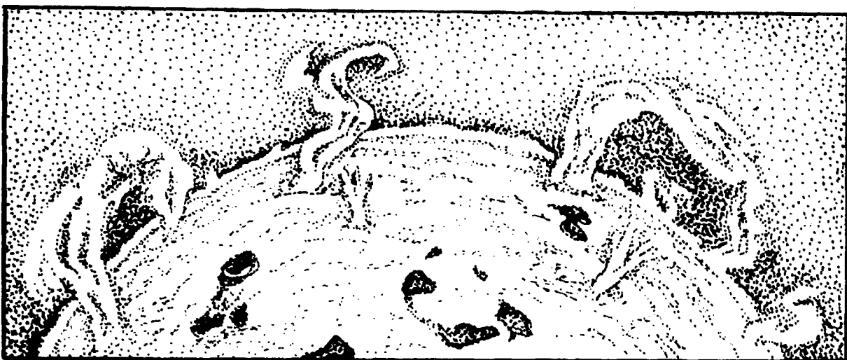
Fig. 9.3. A superfície do Sol está em constante turbulência com fortes correntes de gás e erupções que jogam para a atmosfera solar jatos de gases luminosos (proeminências) que se elevam quilômetros para fora da superfície; algumas manchas solares estão representadas na superfície.
