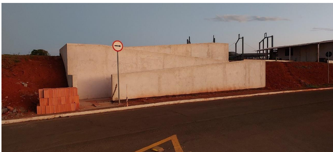
Figura 22 – Detalhe da sinalização podotátil na rampa de transposição de nível entre os prédios 1 (existente) e 2 (em construção)
