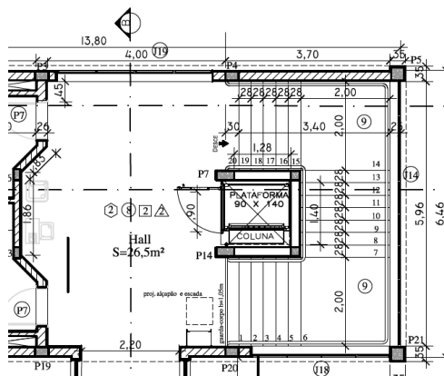
Figura 112 - Plataforma de acesso ao 2º pavimento
