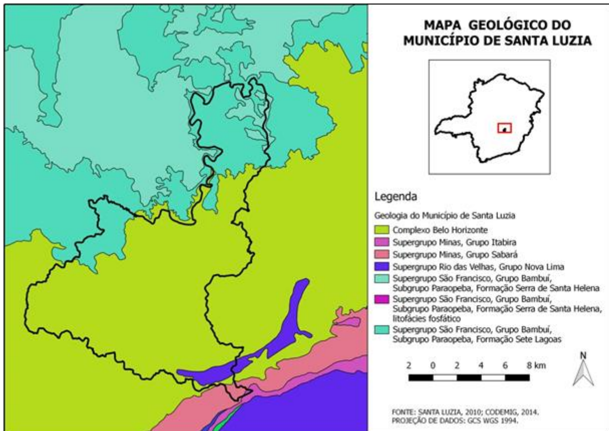
Figura 1 - Mapa geológico do município de Santa Luzia
